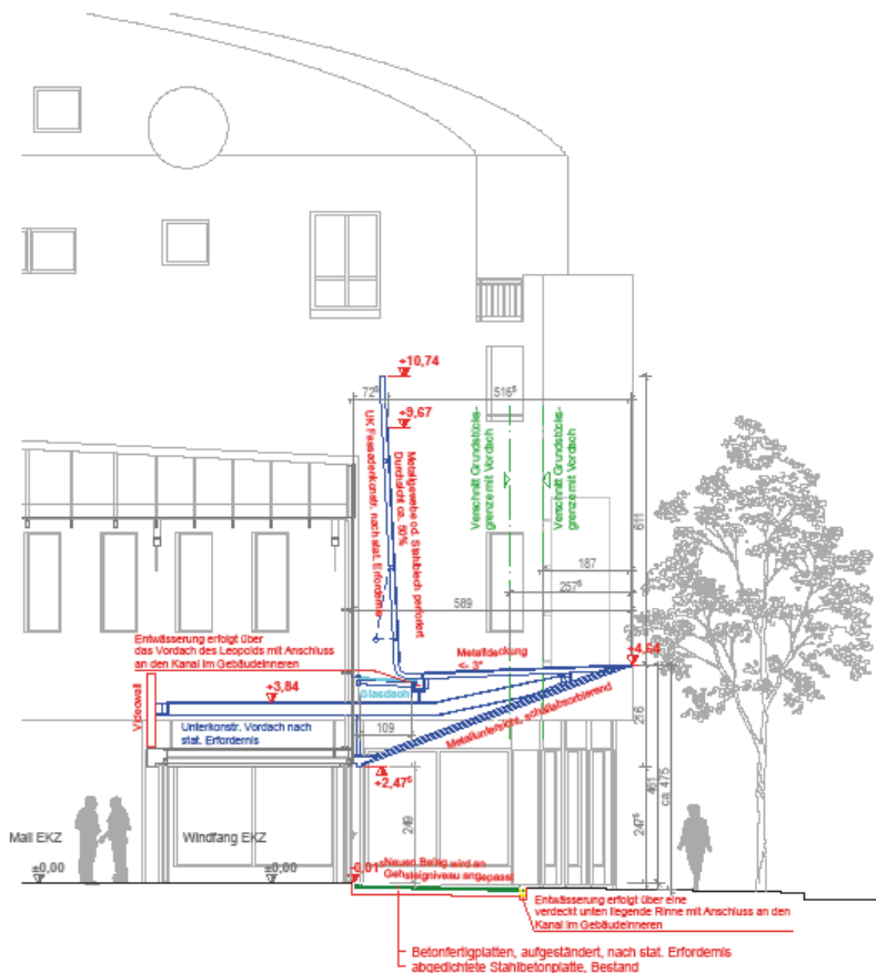
Schnitt 1-1
