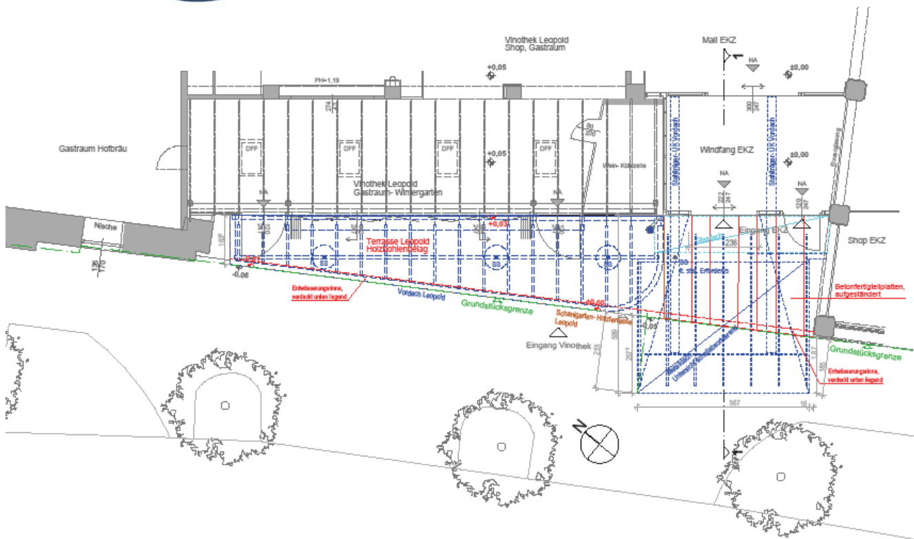
Grundriss
